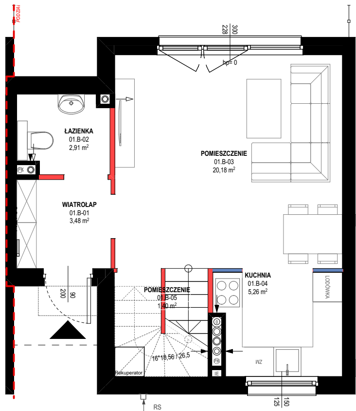
RZUT PARTERU
