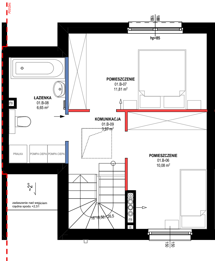
RZUT 1 PIĘTRA
